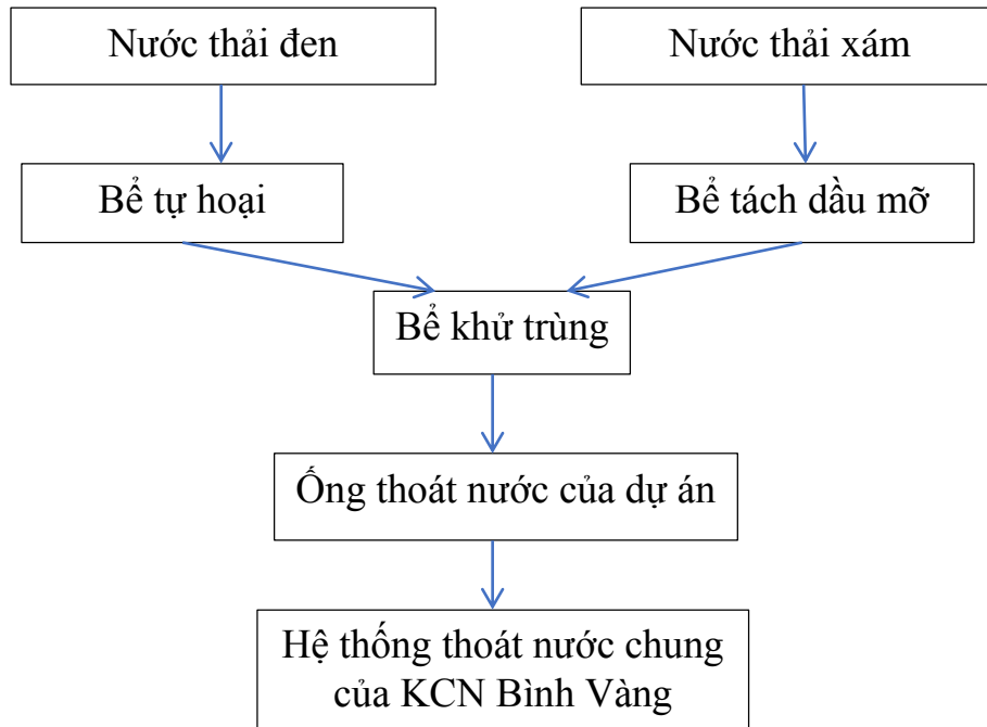
Hình 1. Sơ đồ hệ thống xử lý nước thải sinh hoạt trong giai đoạn vận hành
