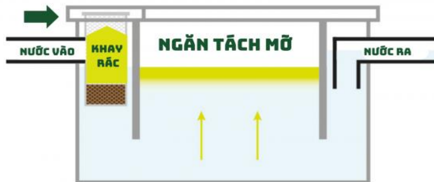
Hình 3. Minh họa nguyên tắc hoạt động của bể tách dầu mỡ
